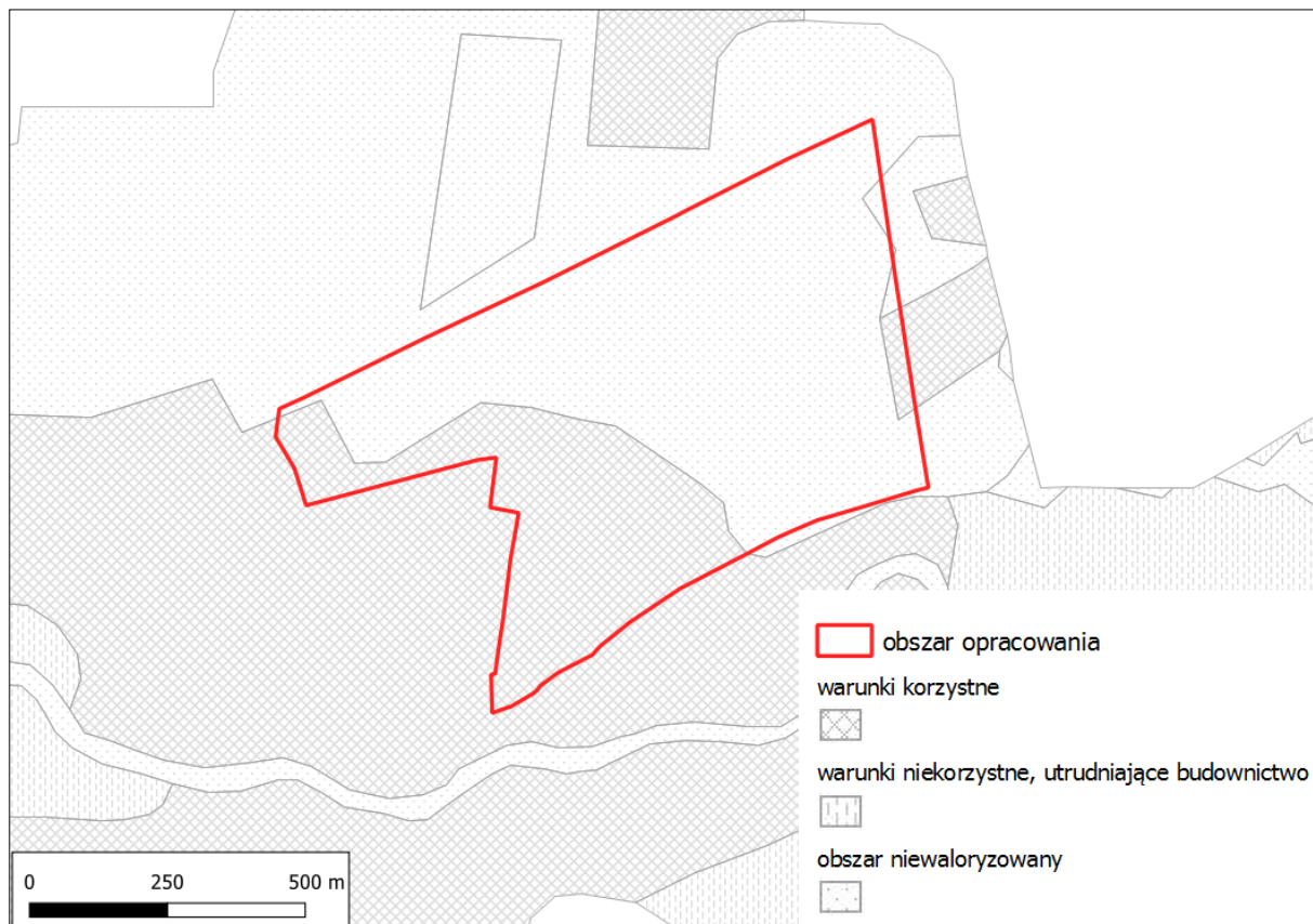
Rysunek 9. Warunki podłoża budowlanego na terenie opracowania Źródło: opracowanie własne na podstawie Mapy geosrodowiskowej Polski 1:50 000
